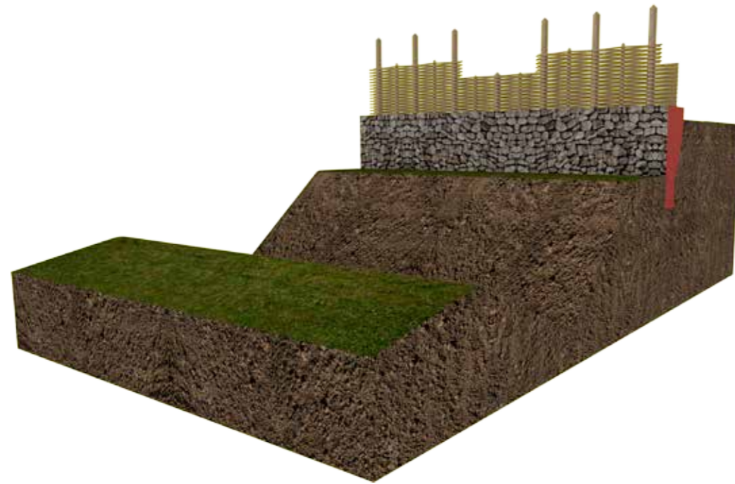
Komplexní opevnění sestávající z ochranného příkopu, kamenné hradby a proplétané palisády
